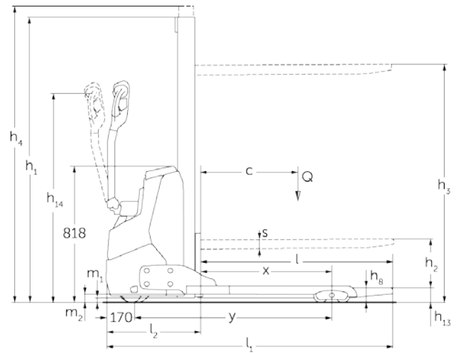
EJC 110bi (Straddle)
